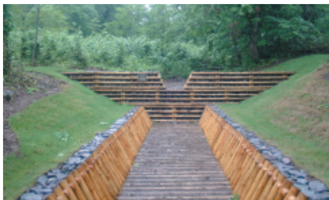
■ 堰堤工・三面張流路工
